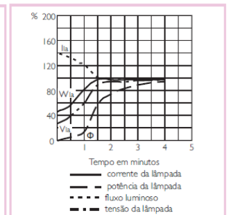
Comportamento da lâmpada durante a partida
