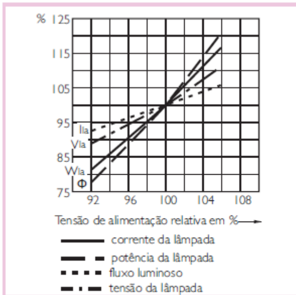
Efeitos de variação da tensão da rede
