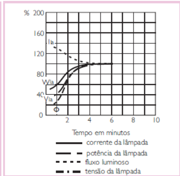
Comportamento da lâmpada durante a partida
