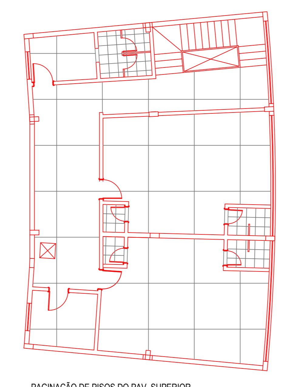
PAGINAÇÃO DE PISOS DO PAV. SUPERIOR
