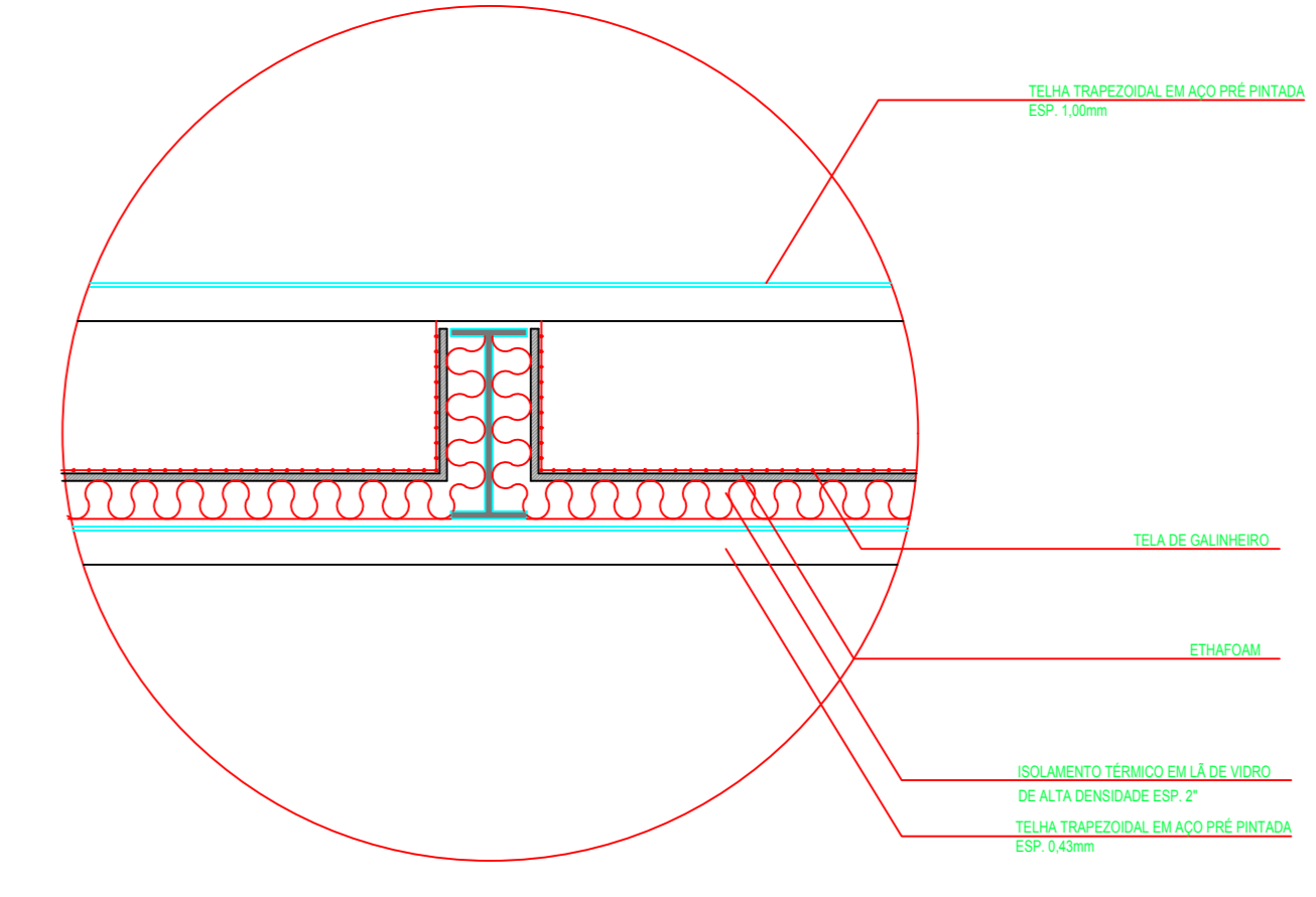
DETALHE DE ISOLAMENTO ACÚSTICO DA COBERTURA MENSURAL
