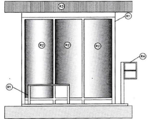
FACHADA Escala 1/20
