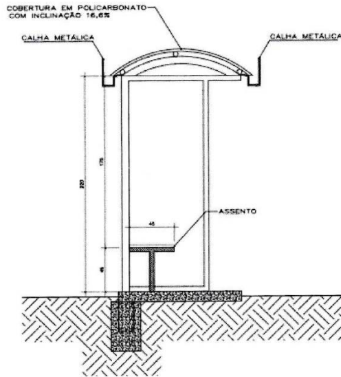
CORTE AA
