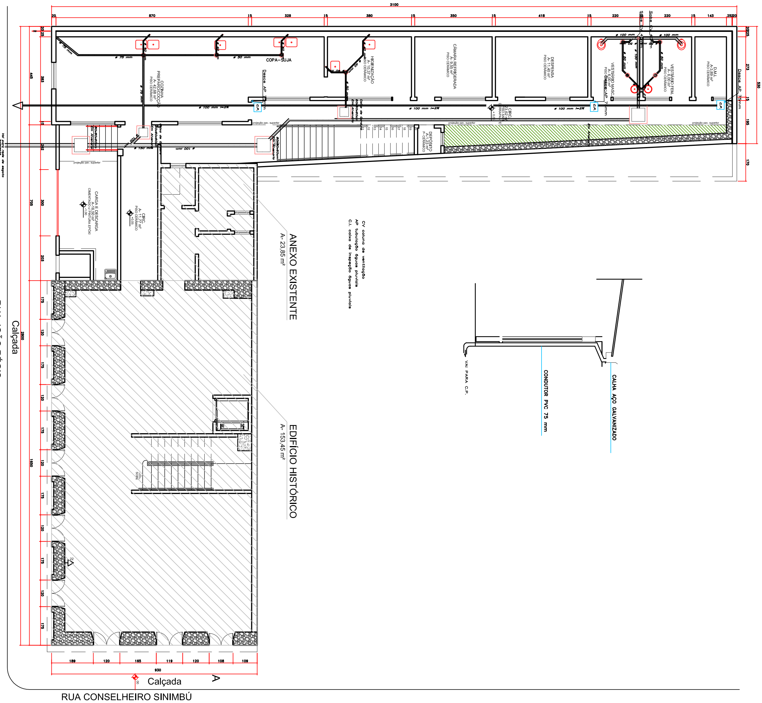
PLANTA TÉRREO
