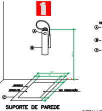
SUPOORTE DE PAREDE DETALHE INSTALAÇÃO DOS EXTINTORES
