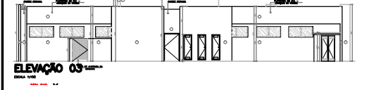
ELEVACÃO 03 ESCALA 1:100
