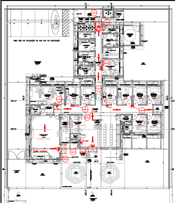
PLANTA BAIXA - USF 2 ESCALA 1:100
