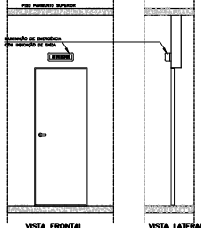
VISTA FRONTAL DETALHE DA INDICAÇÃO LUMINOSA DE SAÍDA
