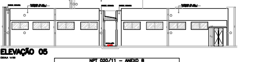
ELEVACÃO 05 ESCALA 1:100
