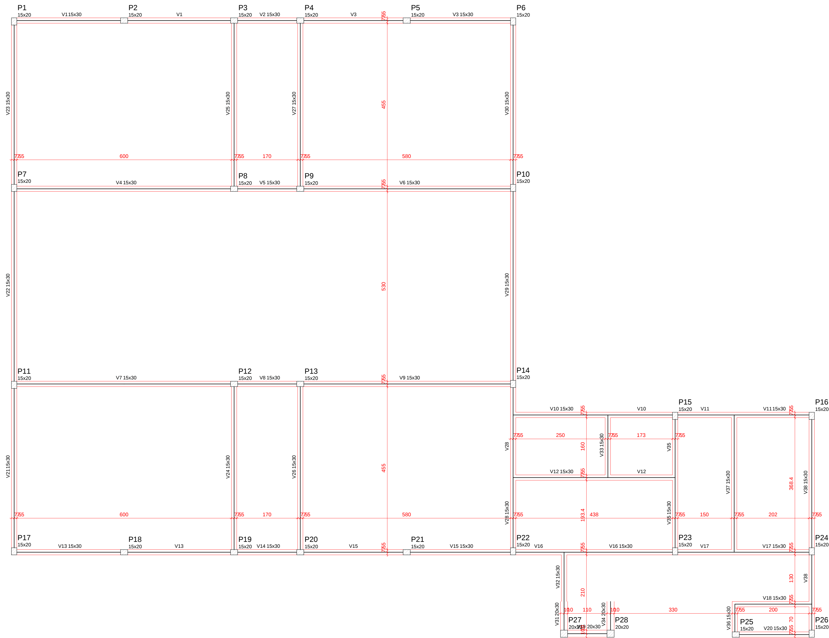
Forma do pavimento Baldrame escala 1:50
