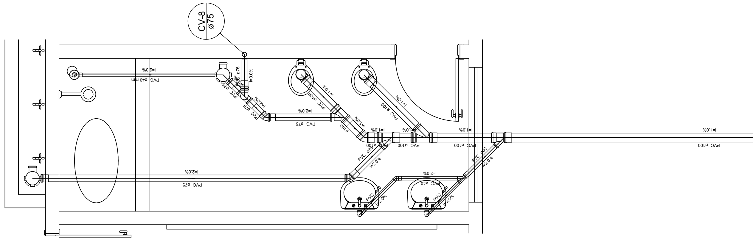
Detalhe S7 escala 1:25
