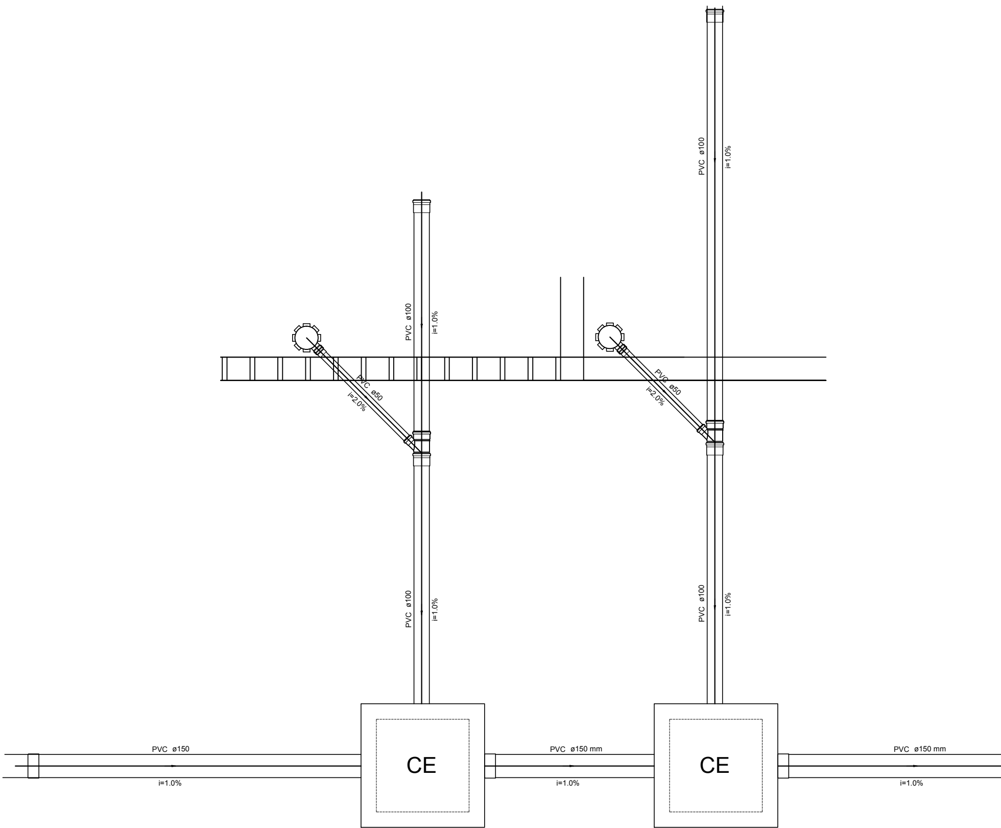
Detalhe S9 escala 1:25
