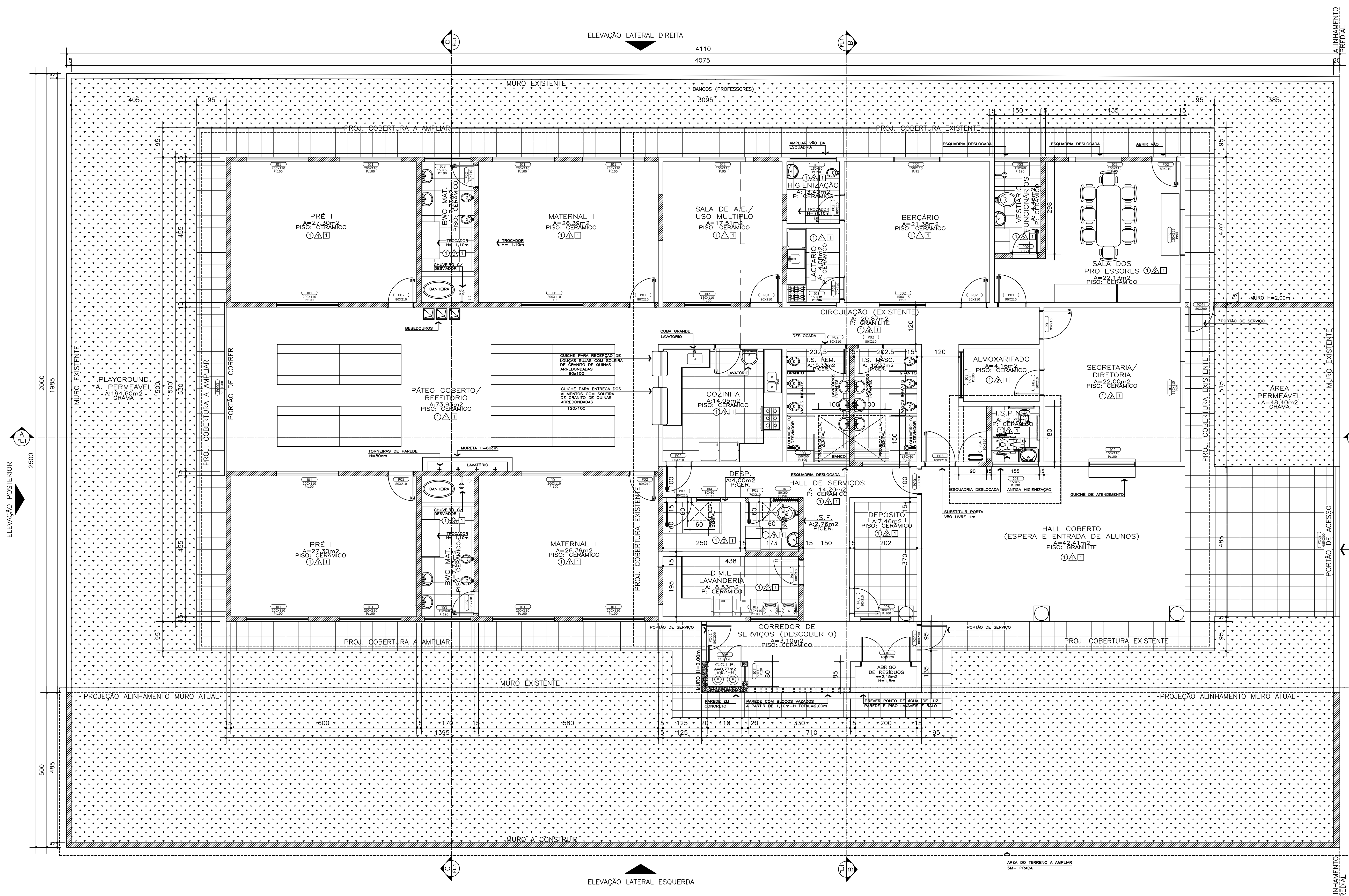
PLANTA BAUXA- AMPLIAÇÃO E REFORMA ESCALA 1/75
