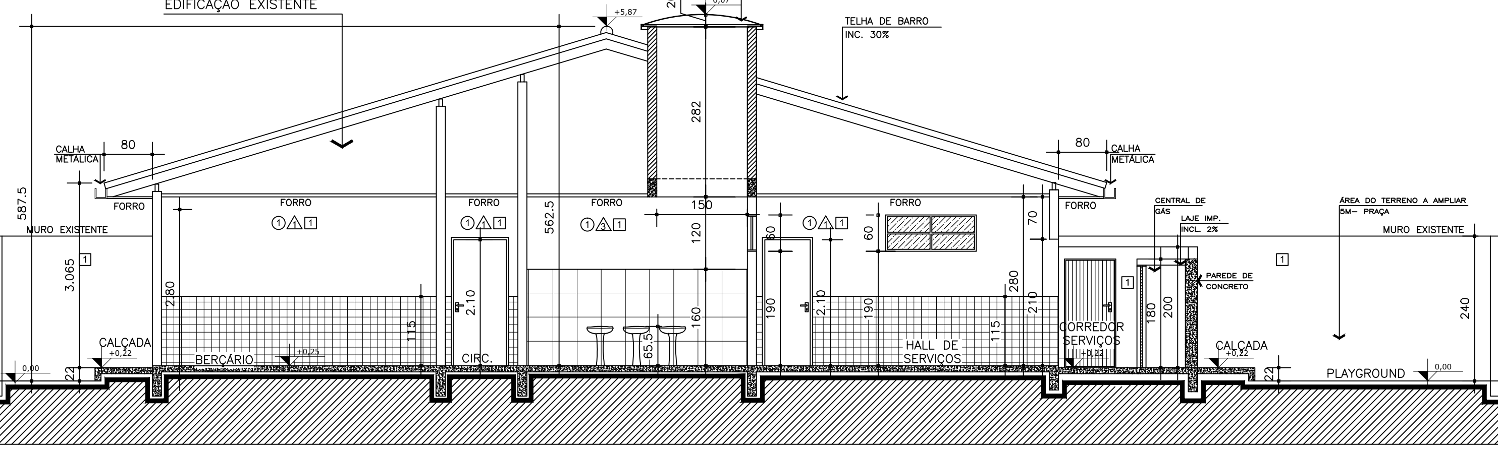
CORTE BB- TRANSVERSAL ESCALA 1/75
