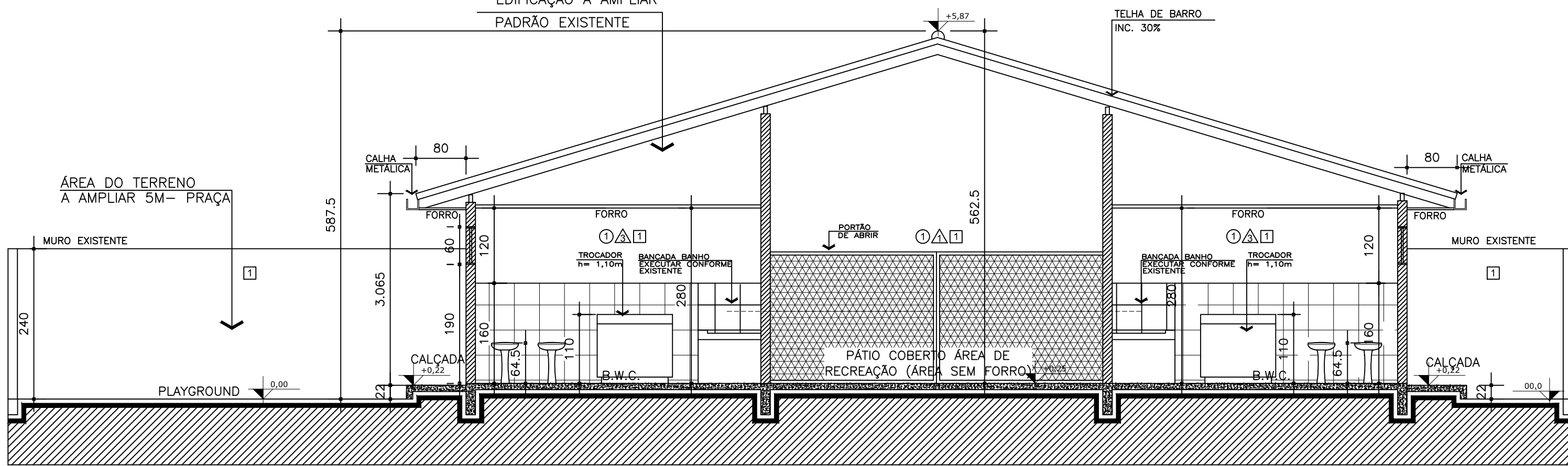
CORTE CC-TRANSVERSAL ESCALA 1/75
