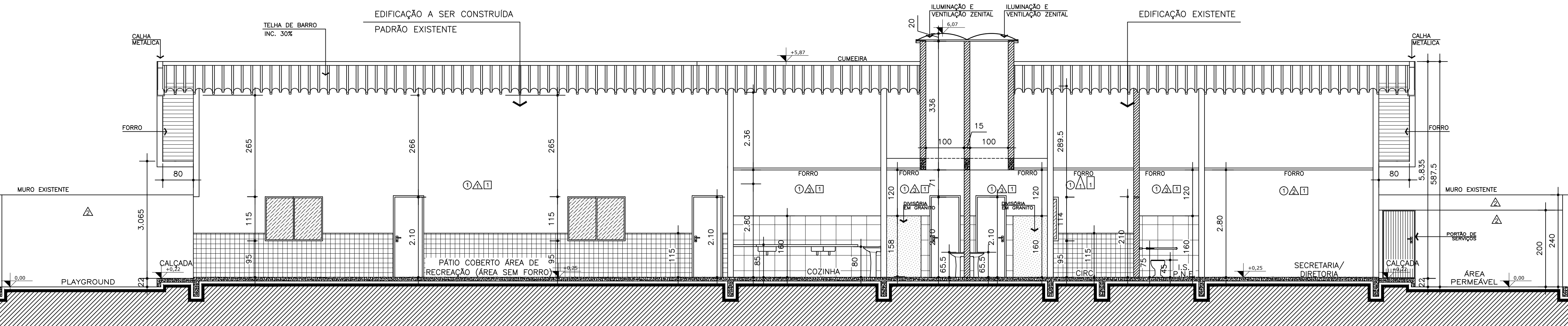
CORTE AA- LONGITUDINAL ESCALA 1/75
