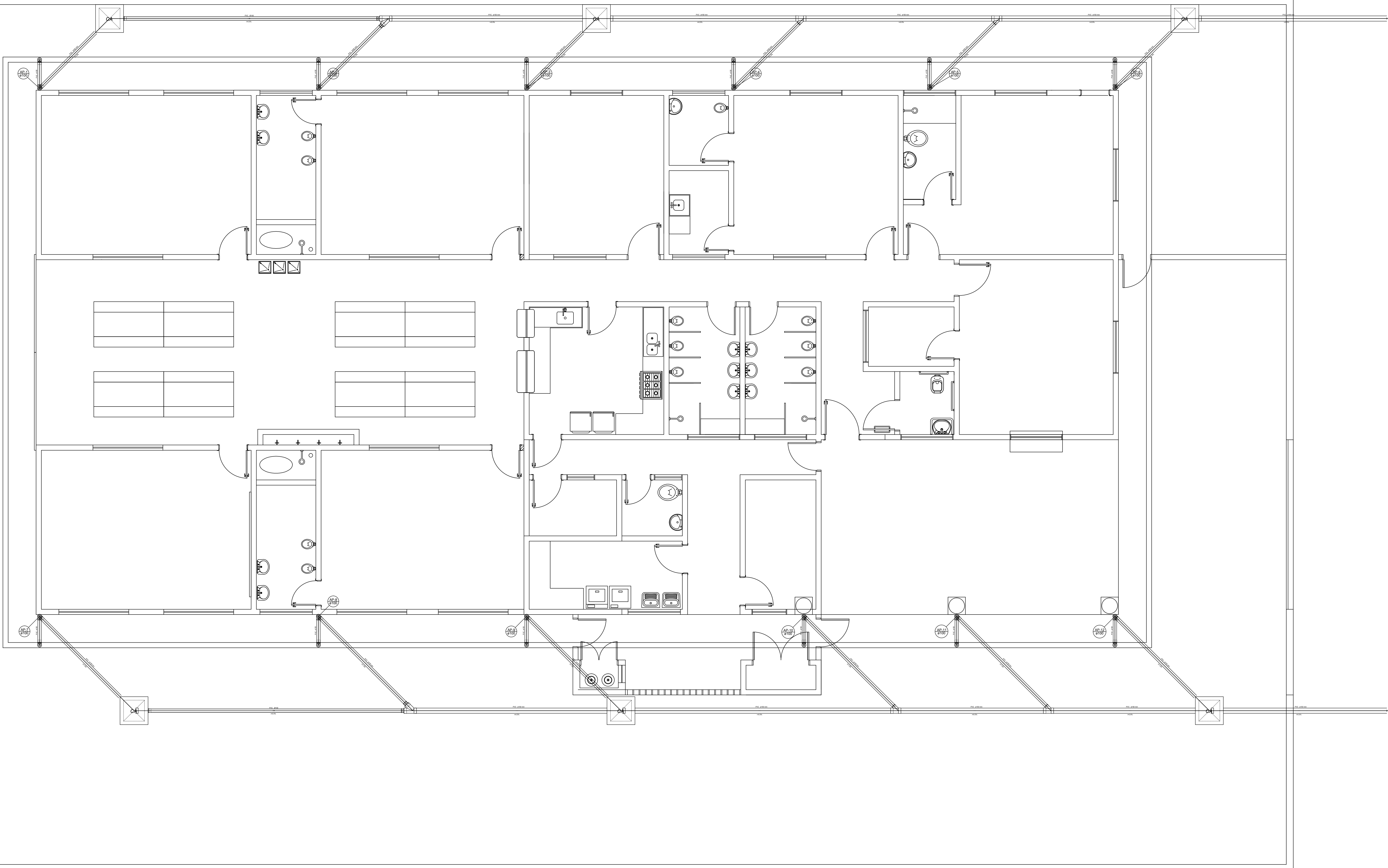
Detalhe S1 escala 1:50
