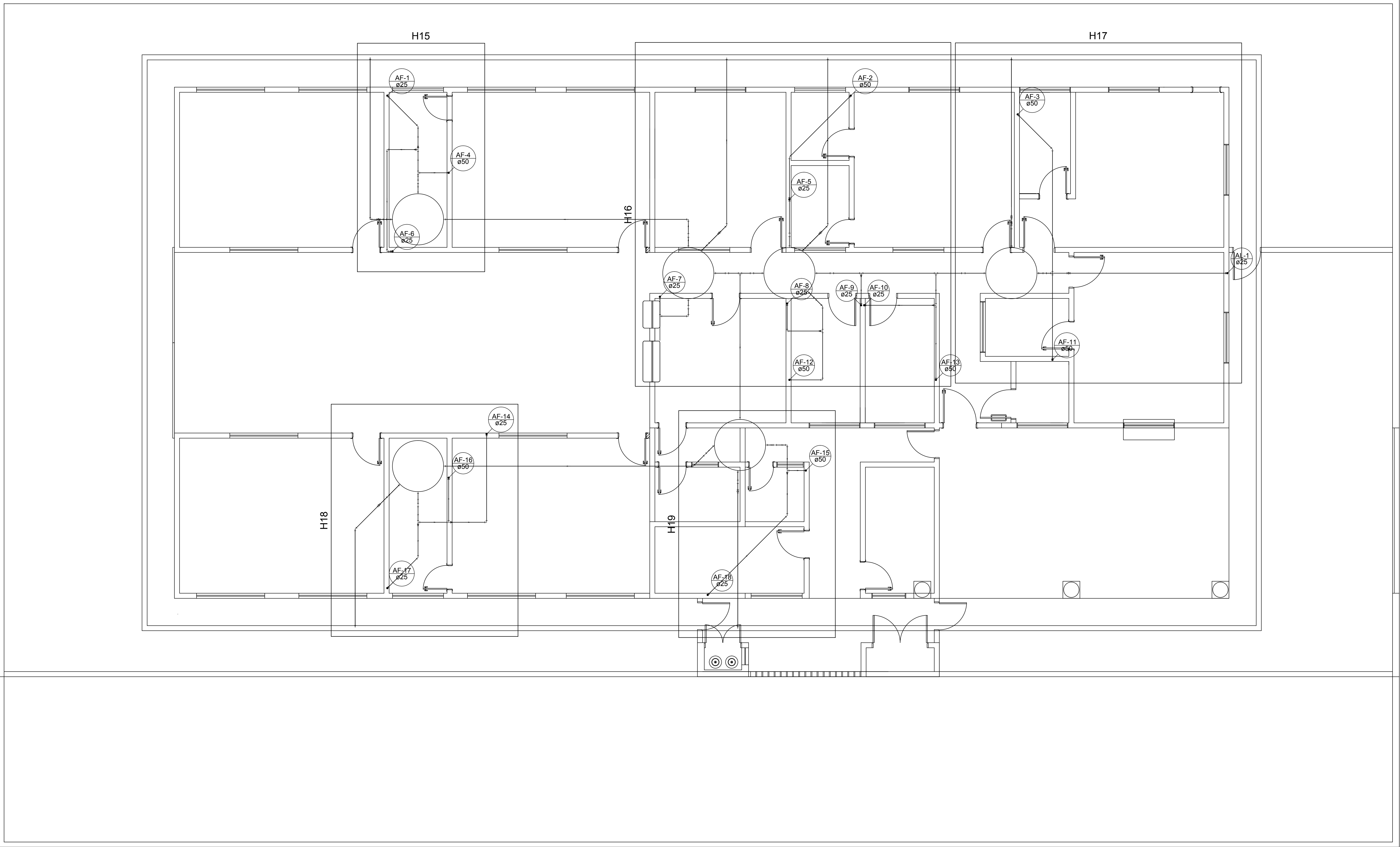
Planta de Cobertura escala 1:50
